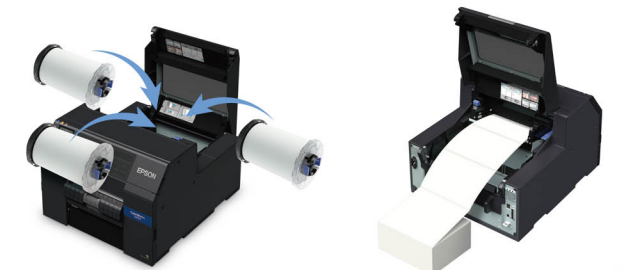
前開蓋
